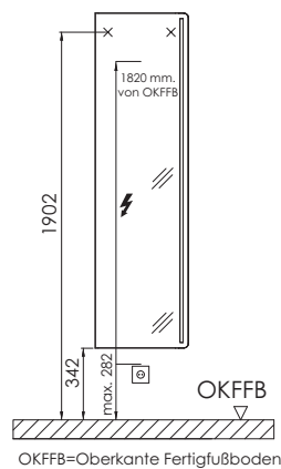
OKFFB=Oberkante Fertigfußboden
