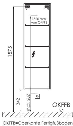
OKFFB=Oberkante Fertigfußboden
